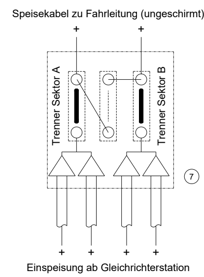
Detail zum Trennkasten
