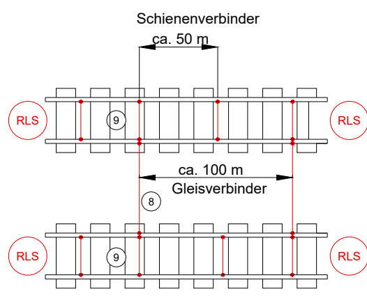
Detail zu Querverbindungen
