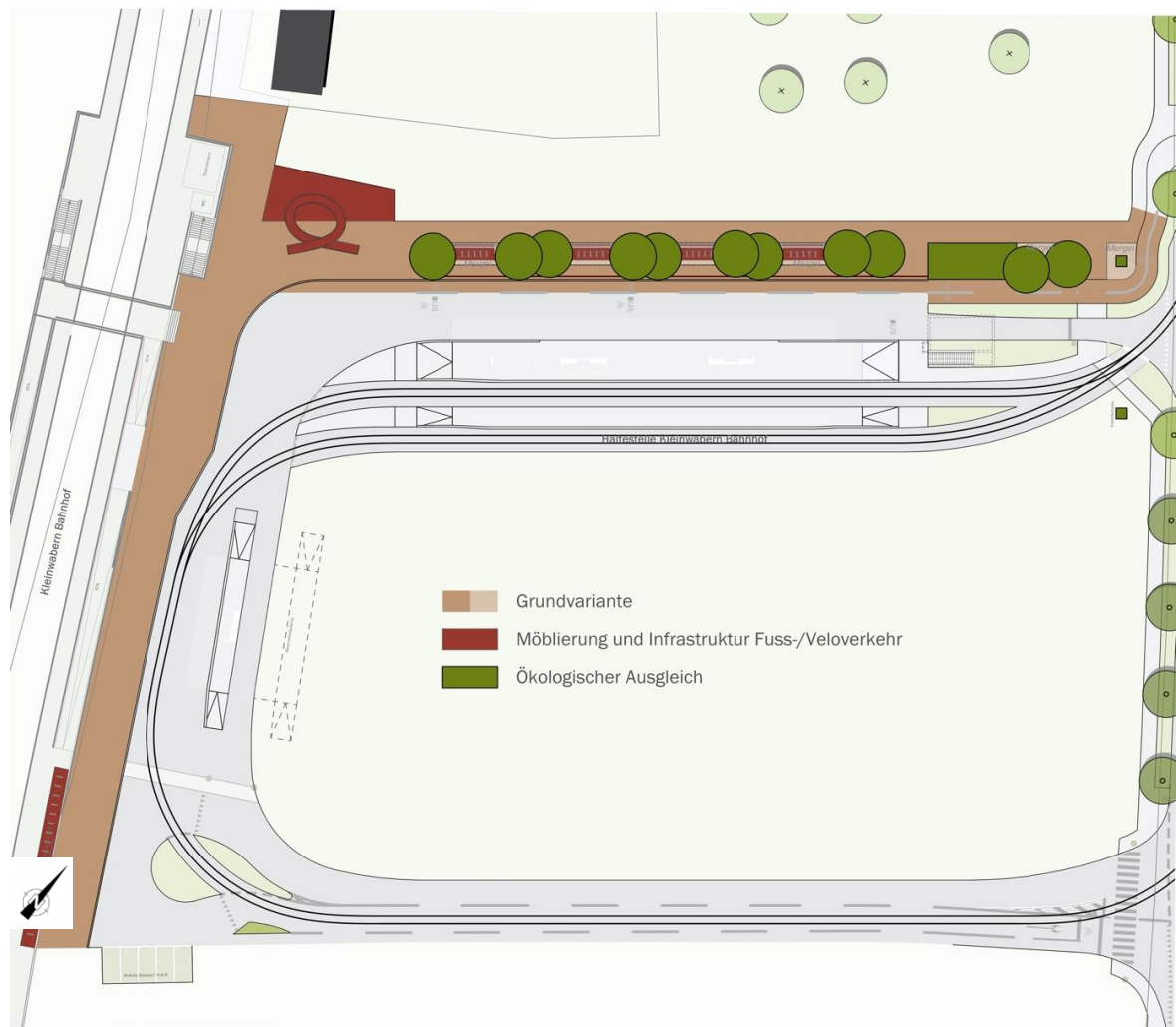
Abbildung 14: Grundausrüstung der Endhaltestelle und Umsteiganlage und Flächen für Möblierung und ökologischen Ausgleich
