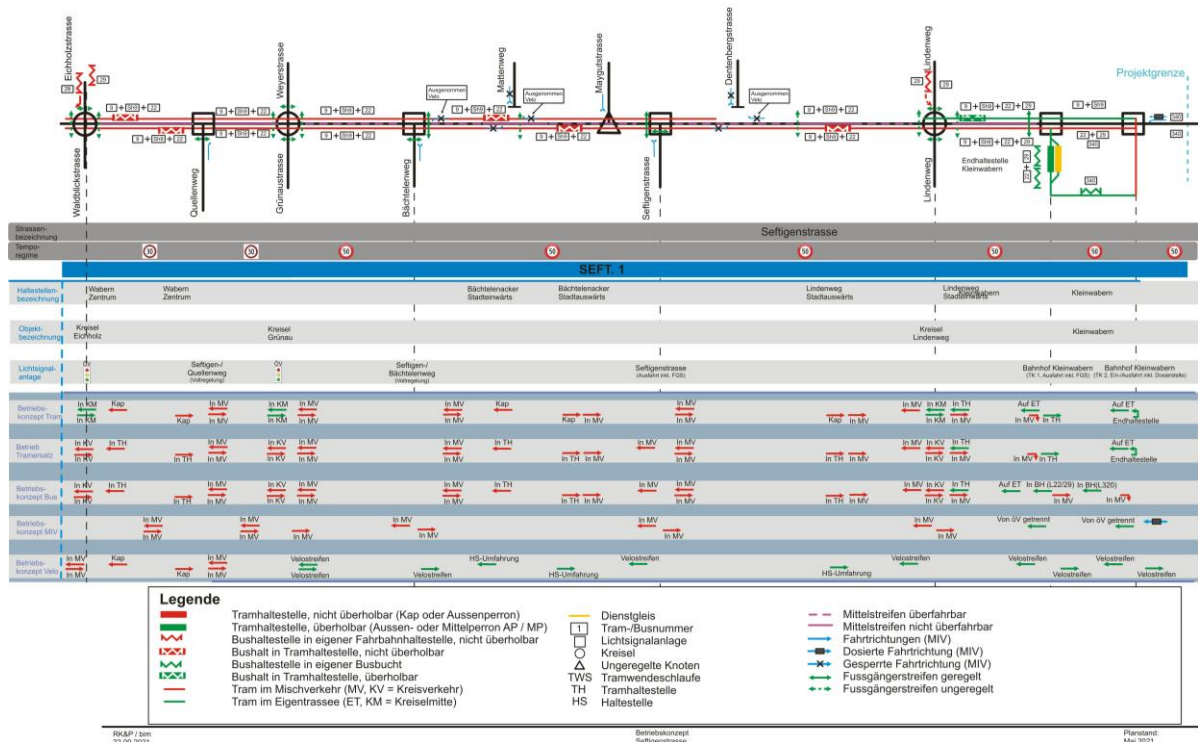
Abbildung 3: Auszug Betriebskonzept Wabern - Kleinwabern (Gesamtplan Nr. SEFT-300 im Dossier)
