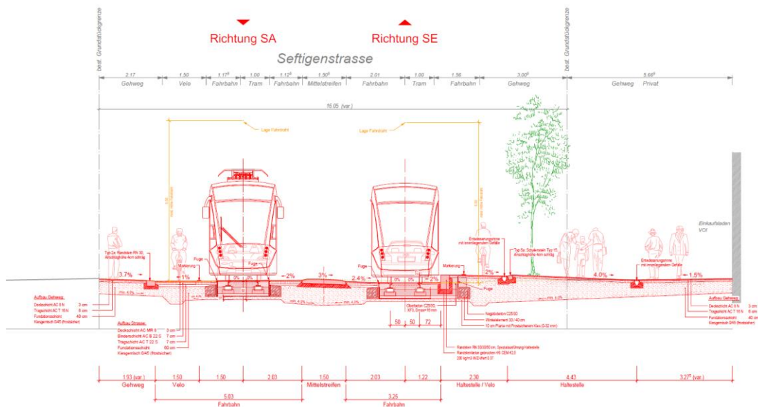
Abbildung 18: Normalprofil Abschnitt 001
