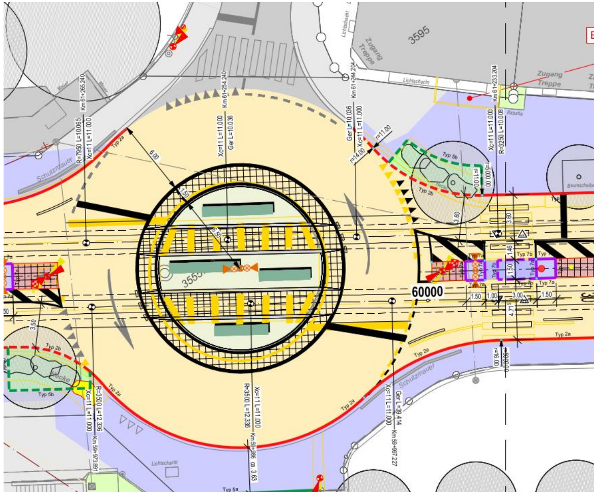
Abbildung 4: Planausschnitt aus Situationsplan. „Kreisel Eichholz - Kreisel Grüнау“
